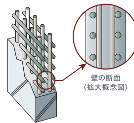
ダブル配筋概念図
