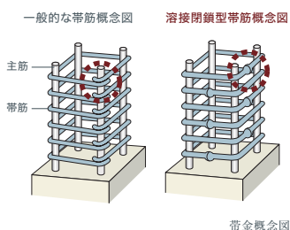
帯筋概念図
