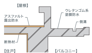
屋上防水対策概念図
