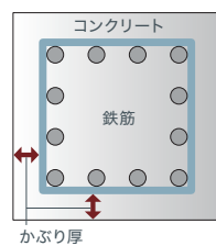
柱の断面概念図
