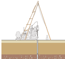
標準貫入試験(機械ボーリング)概略図
