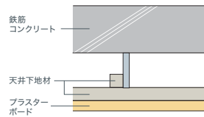
二重天井概念図
